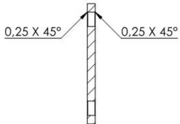
SCHNITT C-C
