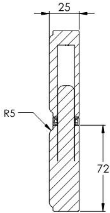
SCHNITT A-A
