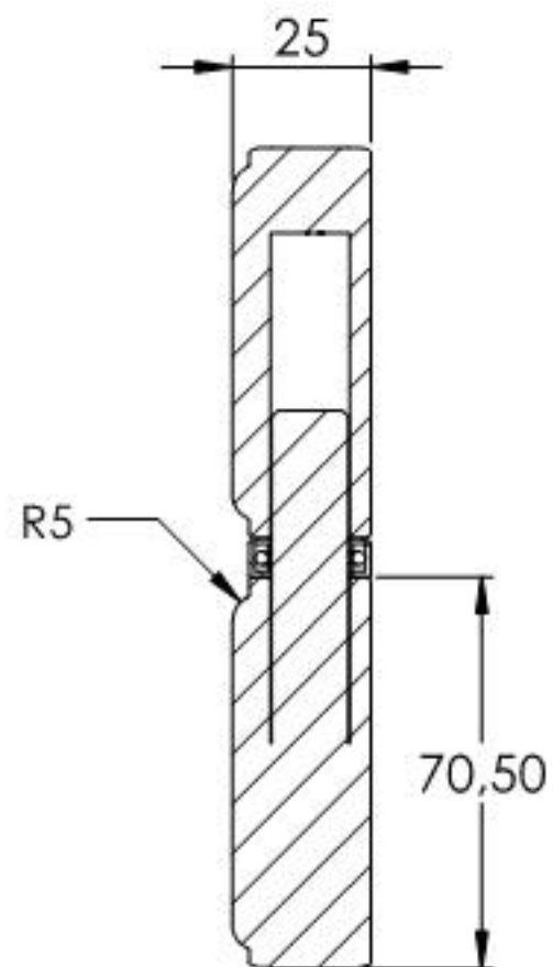
SCHNITT A-A
