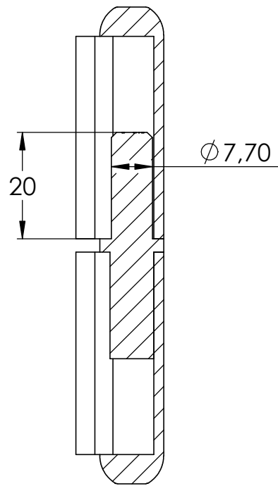
SCHNITT A-A
