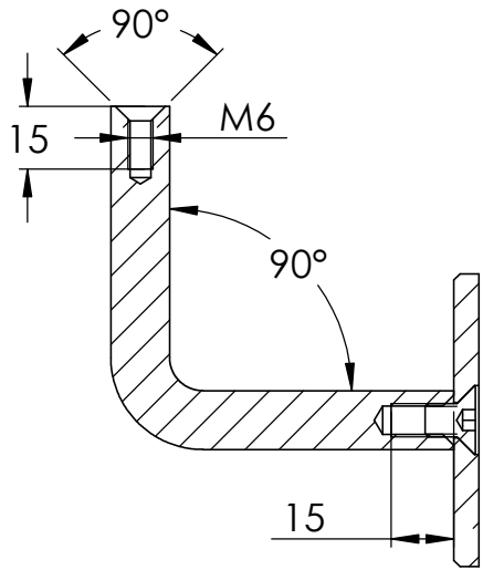
SCHNITT A-A
