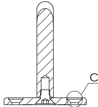
SCHNITT B-B
