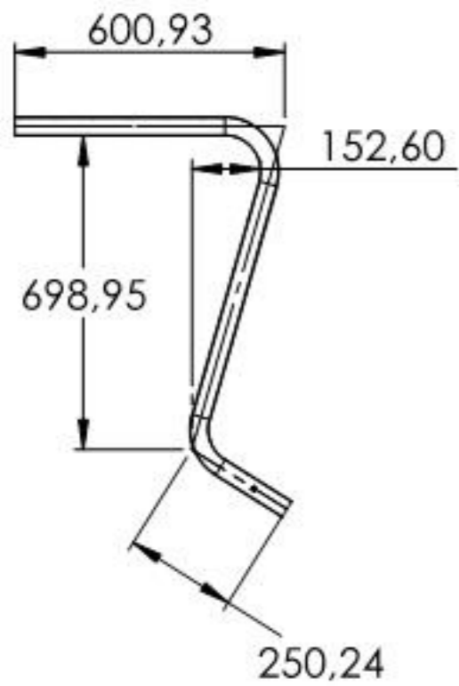
SCHNITT A-A
