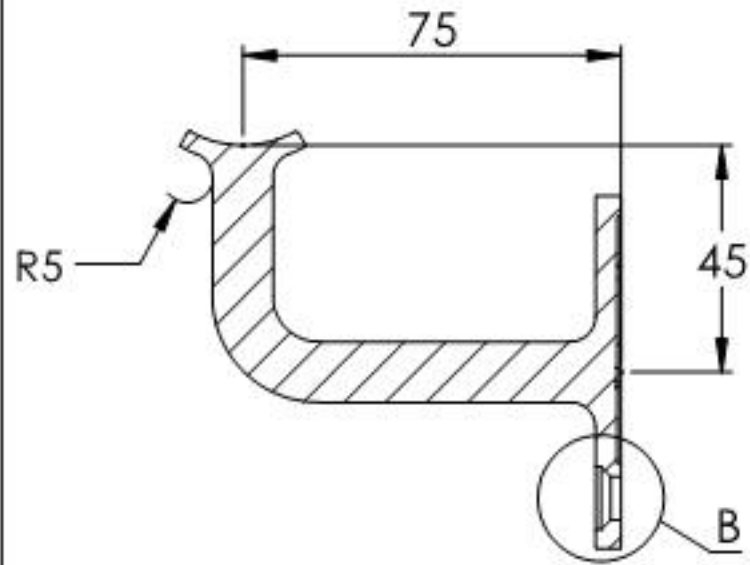
SCHNITT A-A
