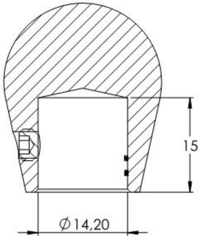
SCHNITT A-A
