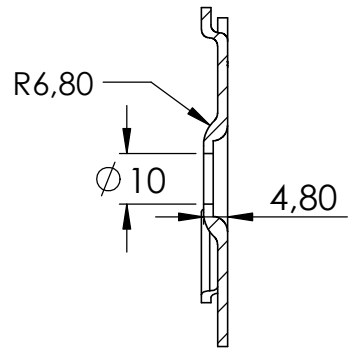
SCHNITT A-A
