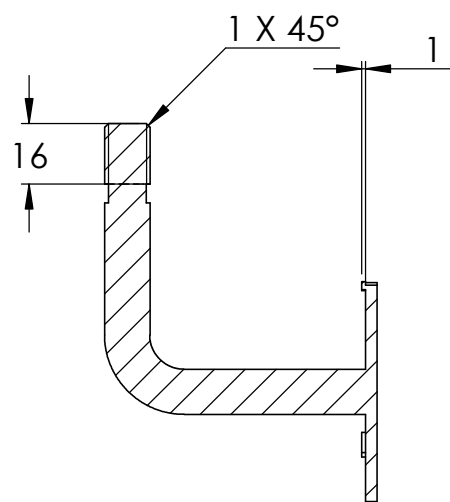
SCHNITT A-A
