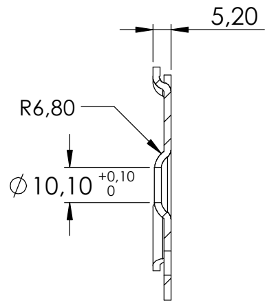
SCHNITT A-A
