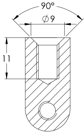
SCHNITT D-D
