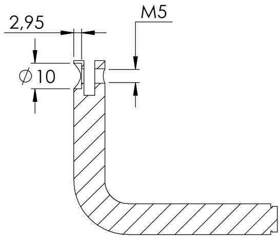
SCHNITT B-B
