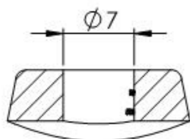
SCHNITT A-A
