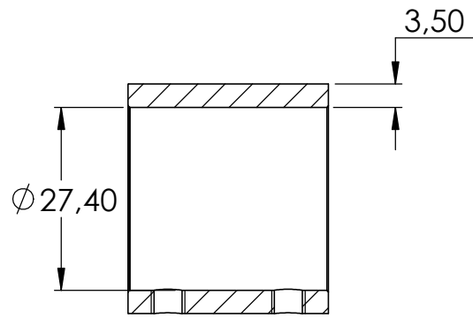
SCHNITT B-B
