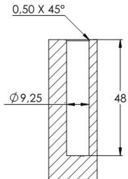
SCHNITT C-C
