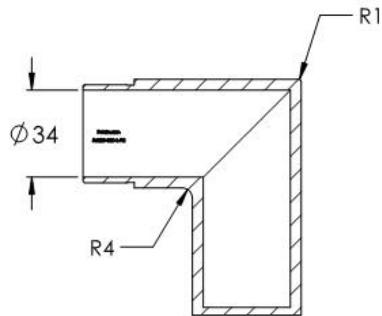
SCHNITT A-A
