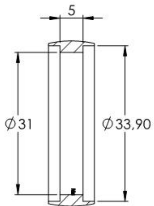
SCHNITT A-A
