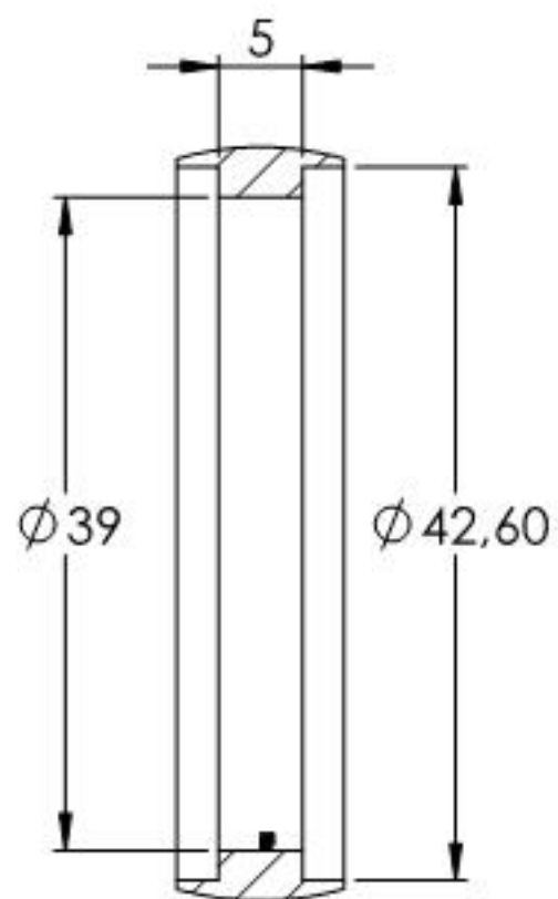
SCHNITT A-A
