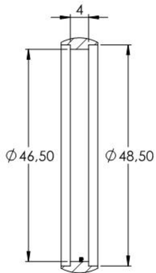
SCHNITT A-A
