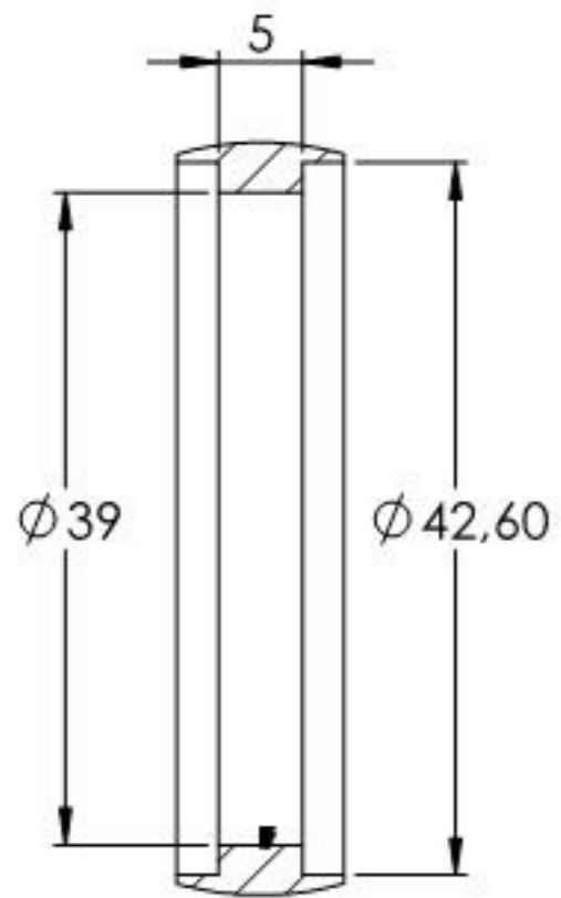
SCHNITT A-A
