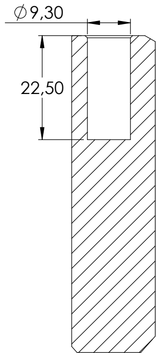
SCHNITT B-B
