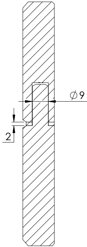
SCHNITT A-A
