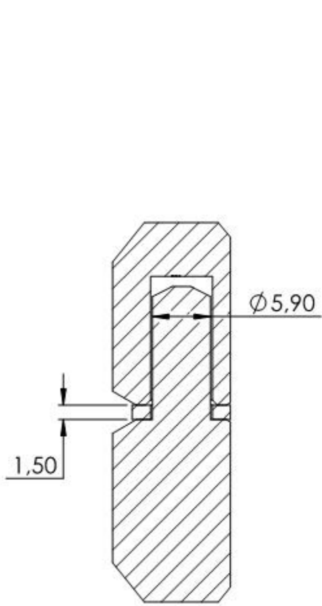
SCHNITT A-A
