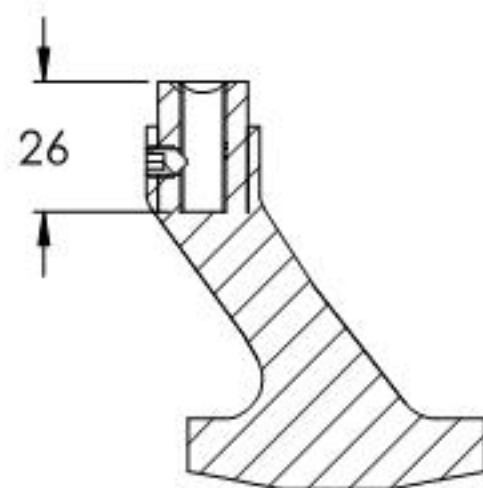
SCHNITT A-A
