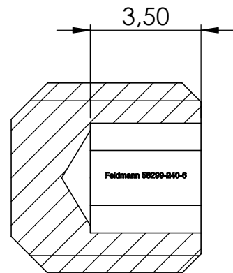
SCHNITT A-A
