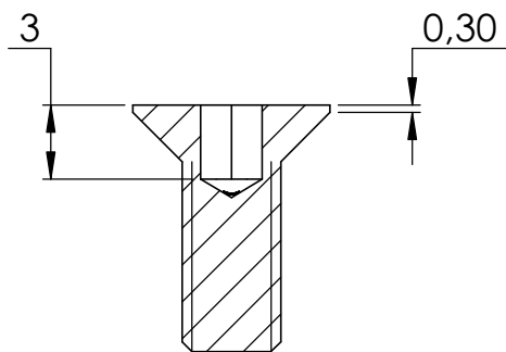
SCHNITT A-A
