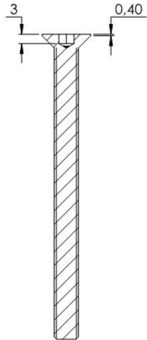
SCHNITT A-A
