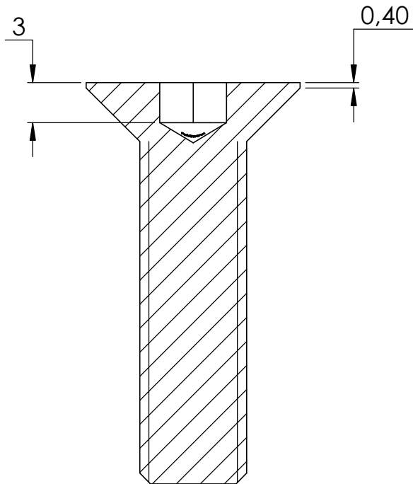
SCHNITT A-A
