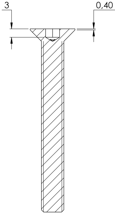
SCHNITT A-A
