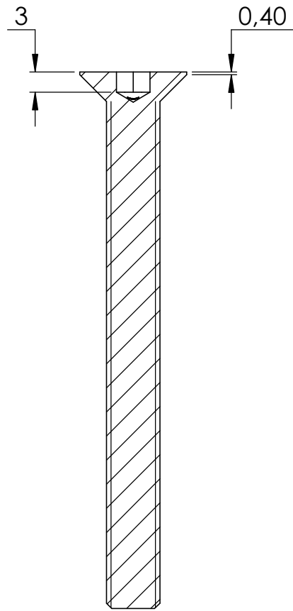
SCHNITT A-A
