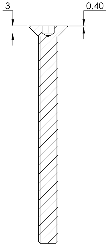
SCHNITT A-A
