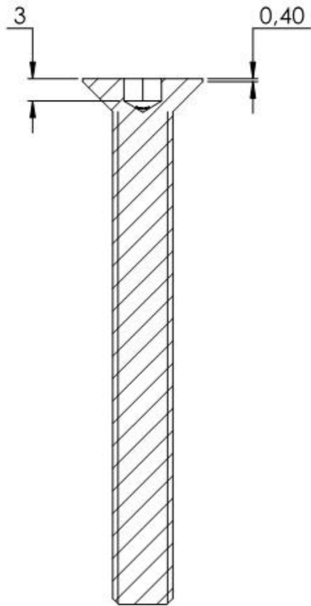
SCHNITT A-A
