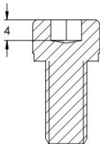
SCHNITT A-A
