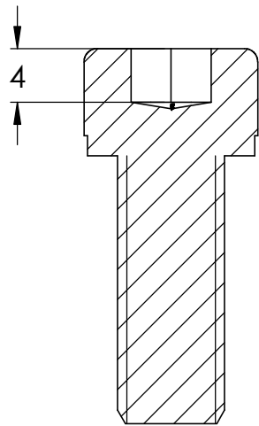
SCHNITT A-A
