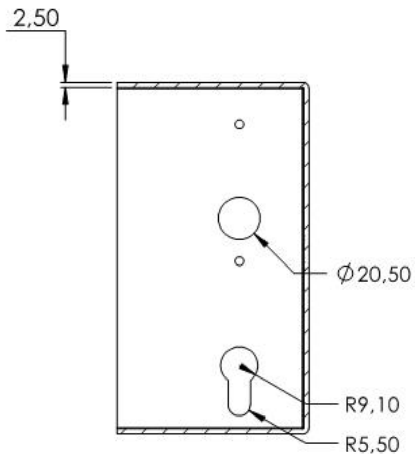
SCHNITT A-A
