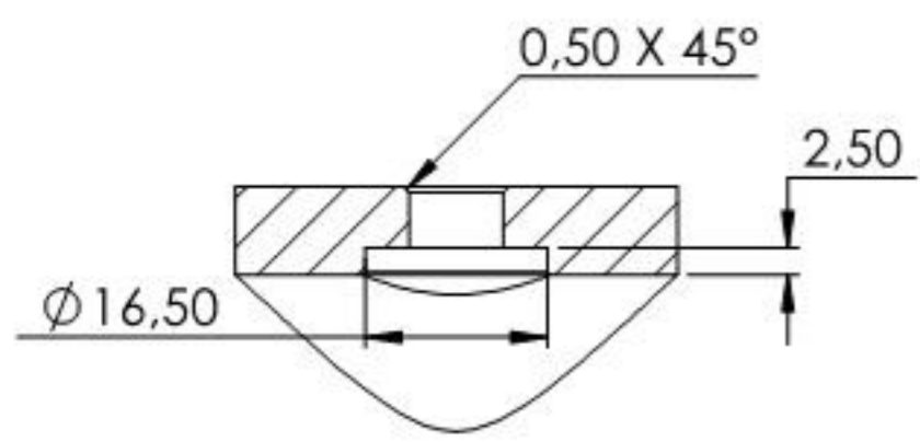
SCHNITT C-C
