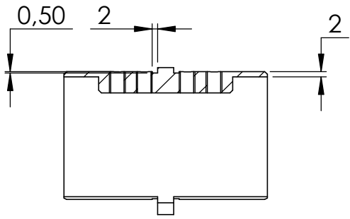
SCHNITT A-A
