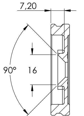
SCHNITT A-A
