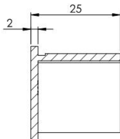
SCHNITT A-A
