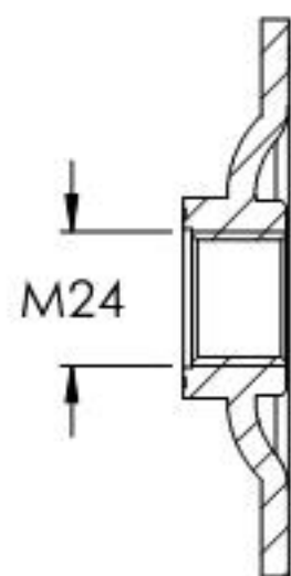
SCHNITT A-A
